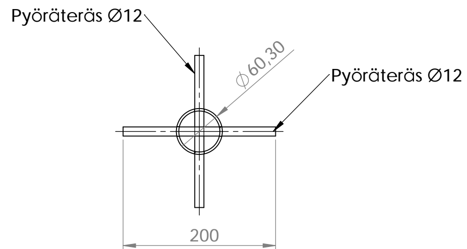
Leikkaus A-A Mitta 1:5
