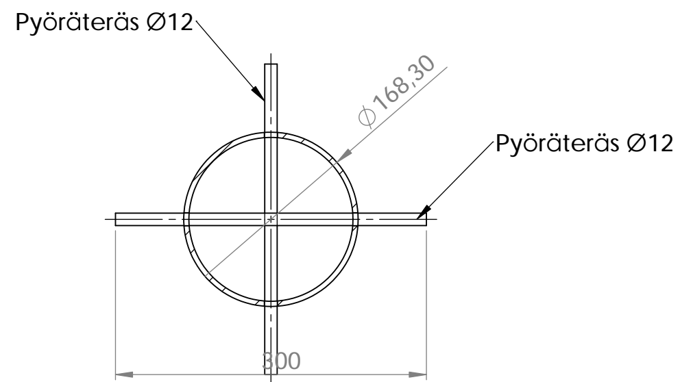
Leikkaus A-A Mitta 1:5
