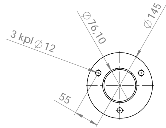
Leikkaus A-A Mitta 1:5
