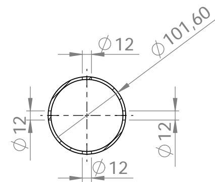
Leikkaus A-A Mitta 1:5
